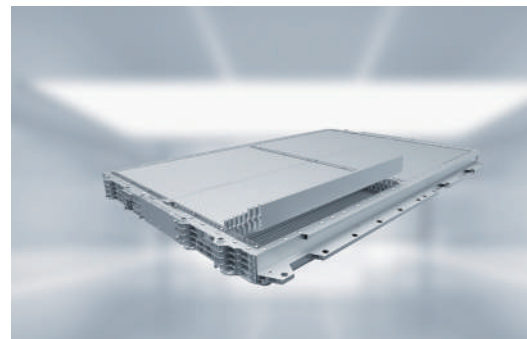
블레이드 배터리 Blade Battery
